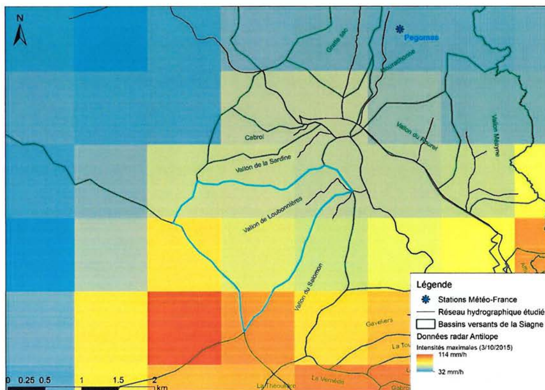
Figure 33 : Pluviométries radar sur le Vallon de Loubonnières et la station Météo-France de Pégomas
