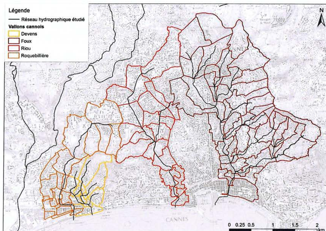
Figure 38 : Bassins versants des vallons cannois faisant l'objet de l'analyse hydrologique
