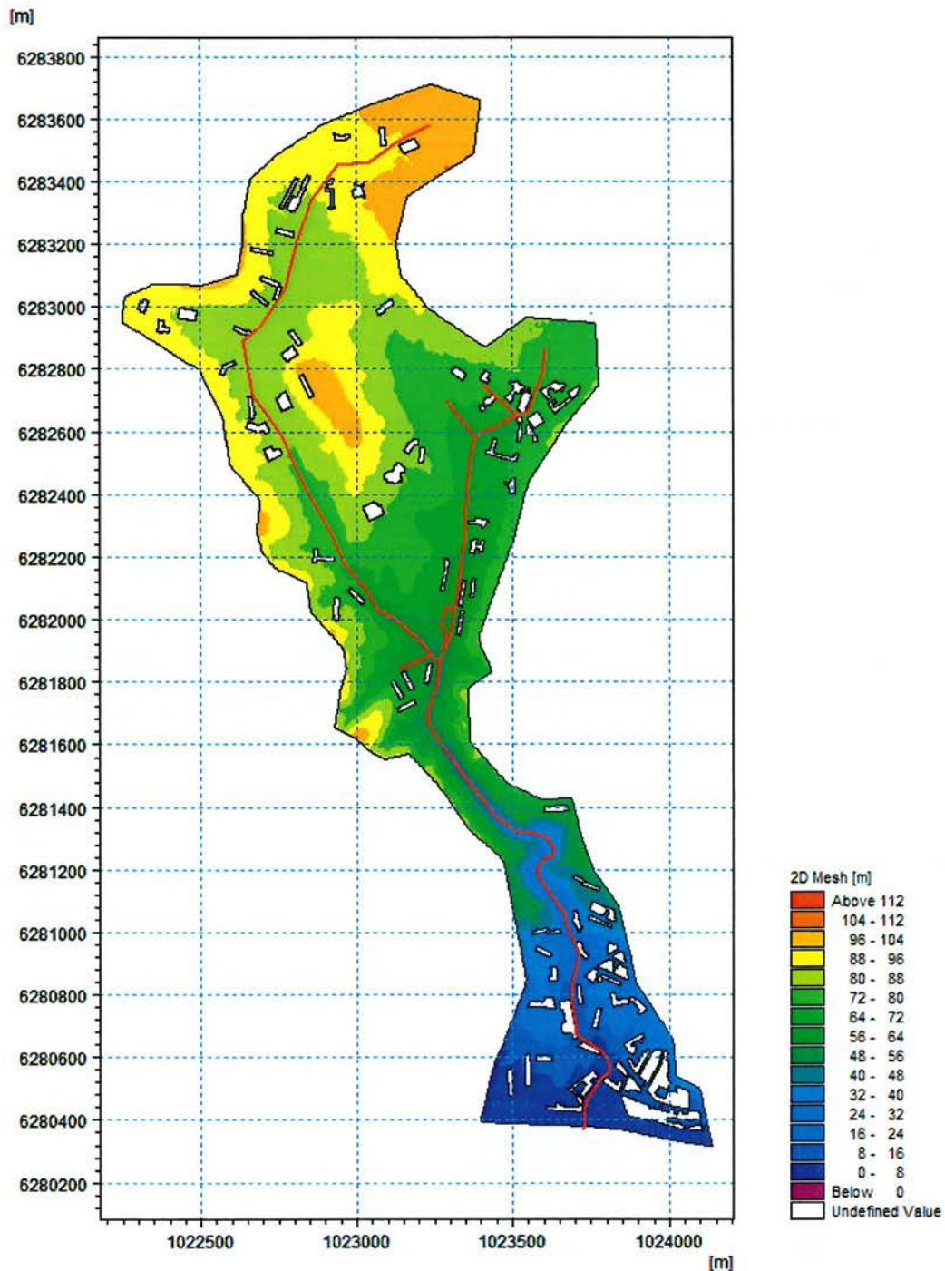
Figure 41 : Vue globale du modèle du vallon du Riou
