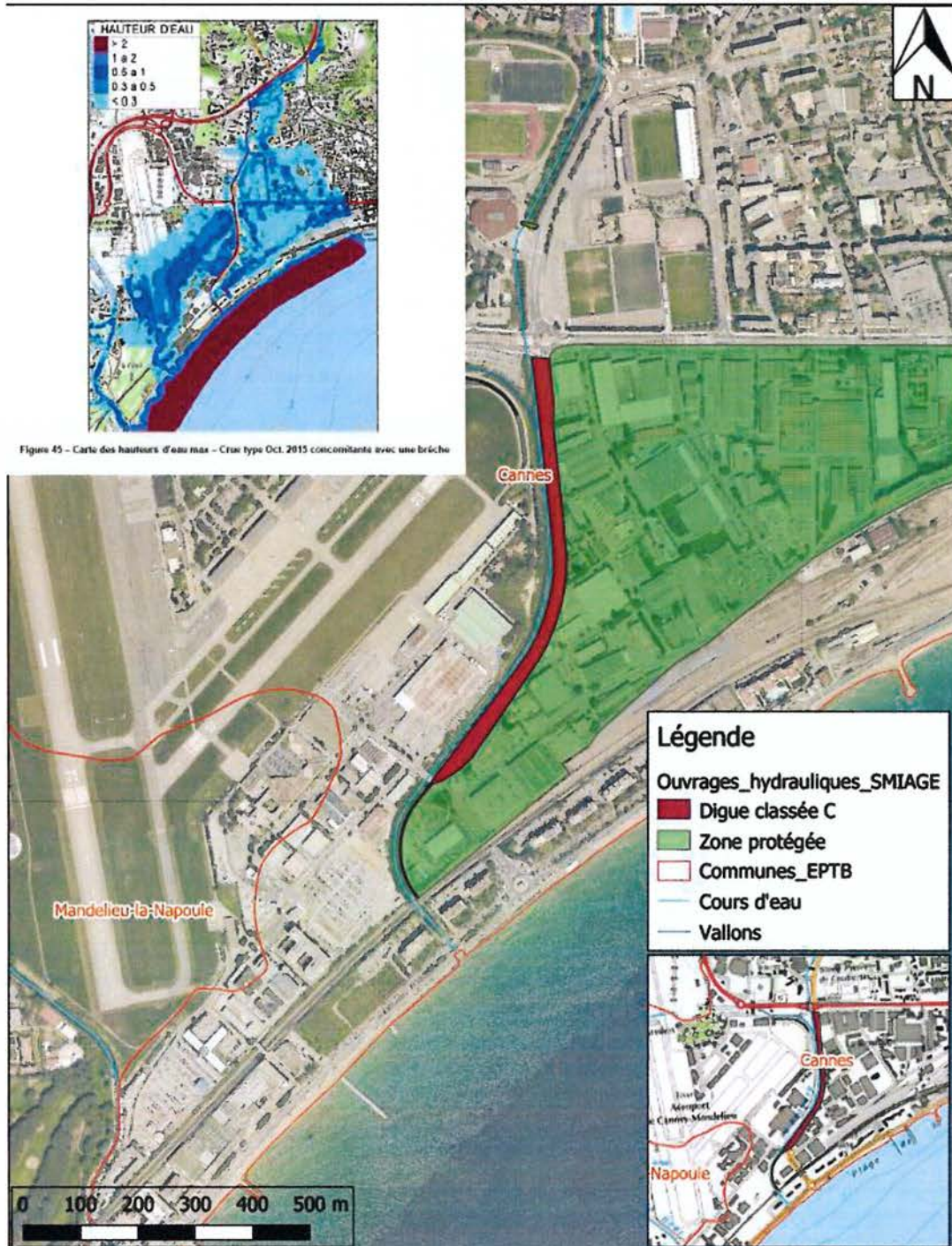
Figure 51 : Localisation de la digue de la Roubine à Cannes
