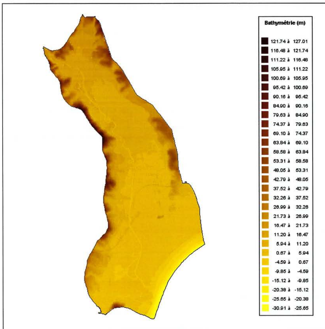
Figure 39 : Vue globale du modèle de la Siagne, du Béal, de la Vieille Siagne, du Gratte-Sac et de la Mourachonne
