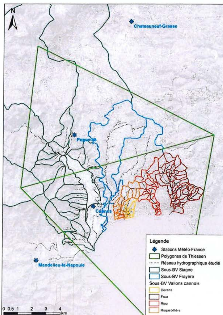
Figure 32 : Affectation des stations pluviométriques à chaque sous-bassin versant
