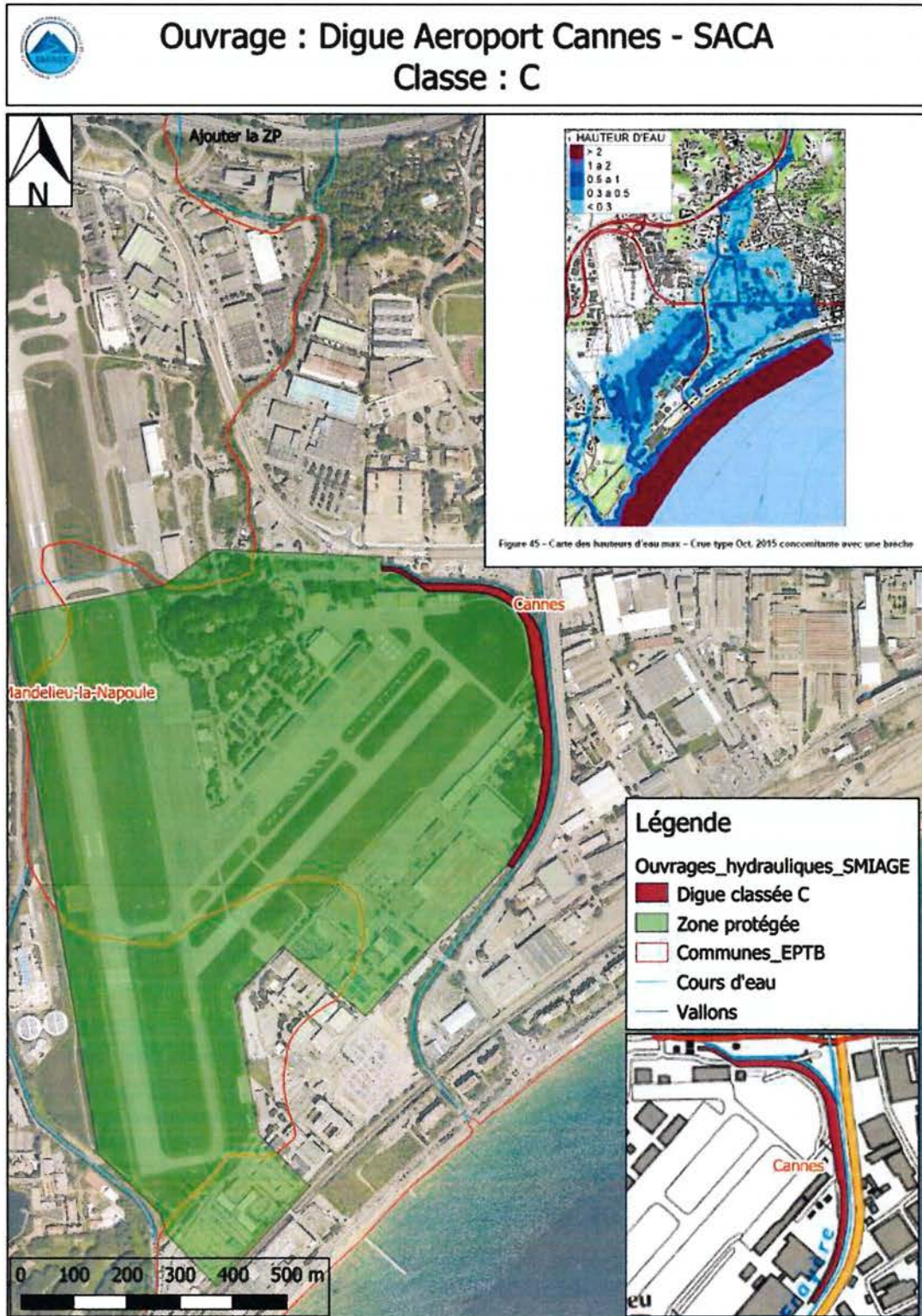
Figure 49 : Localisation de la digue de l'aéroport à Cannes
