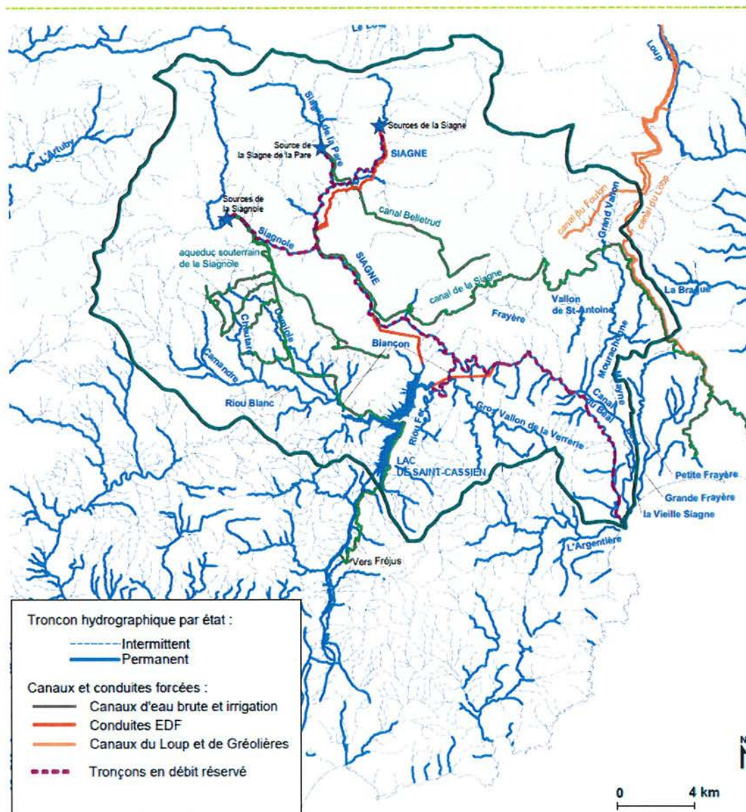
Figure 6 : Réseau hydrographique du bassin versant de la Siagne (Source : SIVU Haute Siagne)
