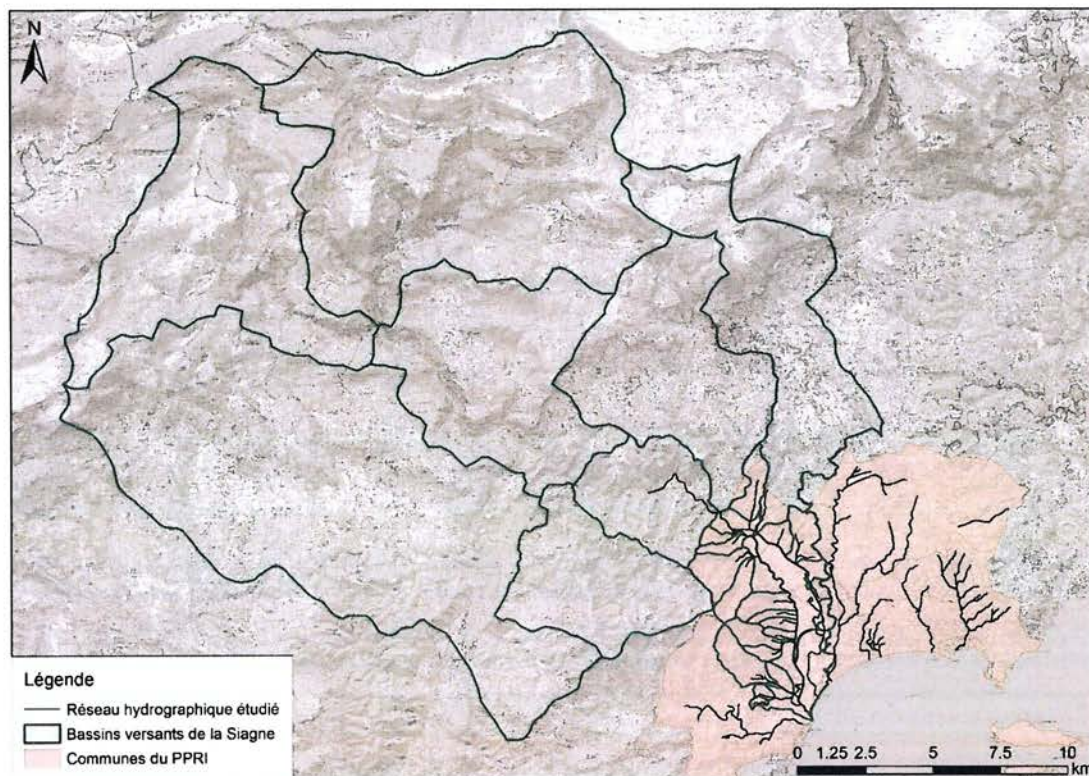
Figure 36 : Bassin versant de la Siagne et ses sous-bassins versants
