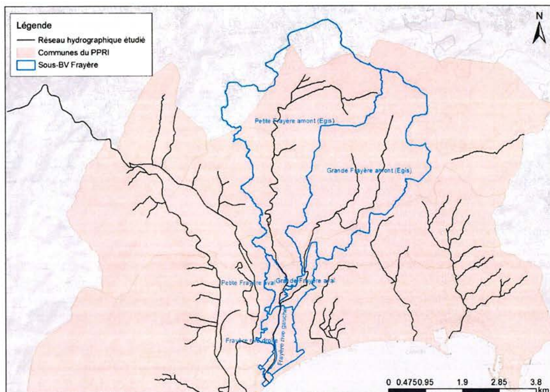
Figure 37 : Bassins versants de la Frayère faisant l'objet de l'analyse hydrologique
