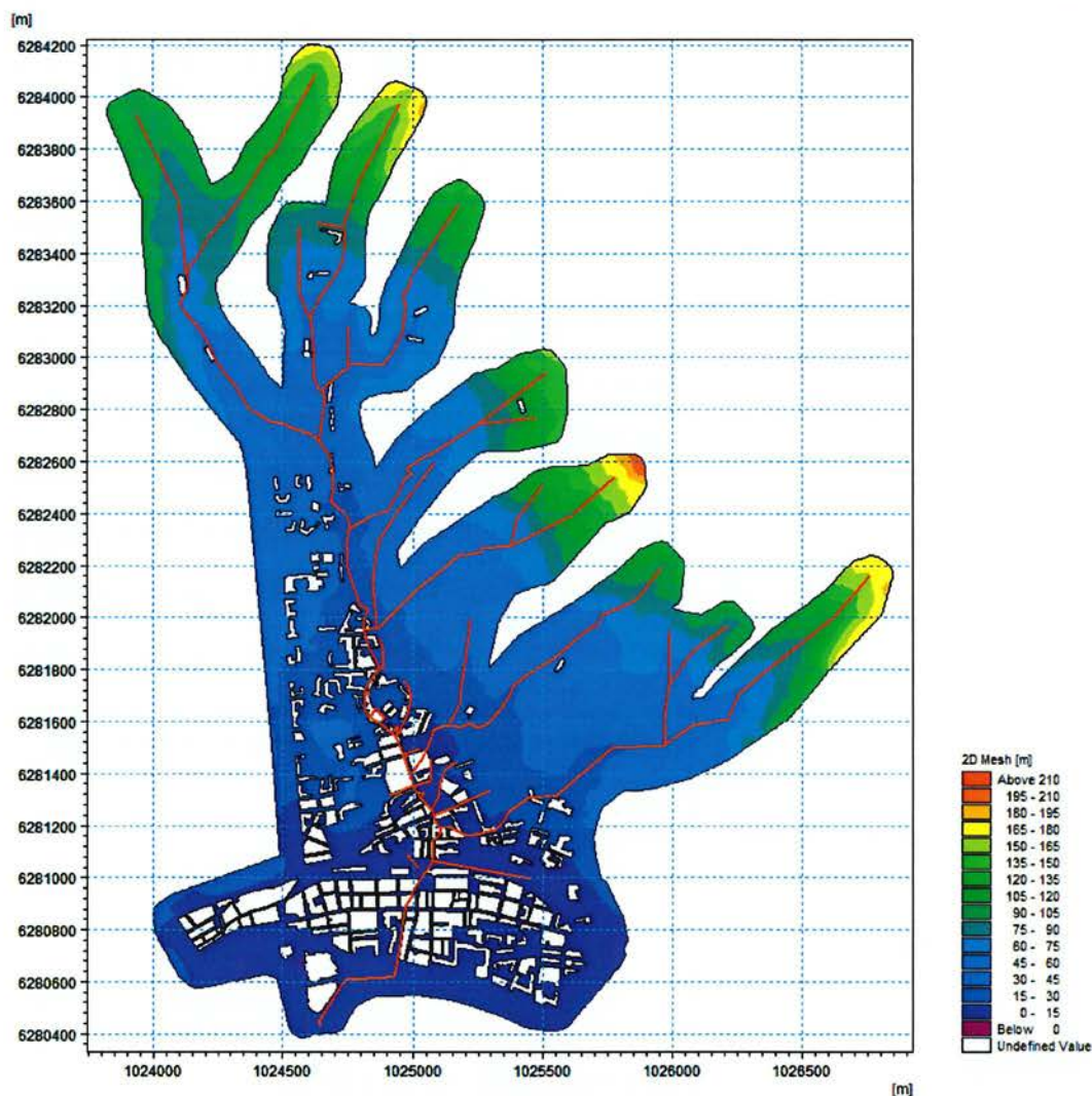
Figure 42 : Vue globale du modèle du vallon de la Foux et ses affluents
