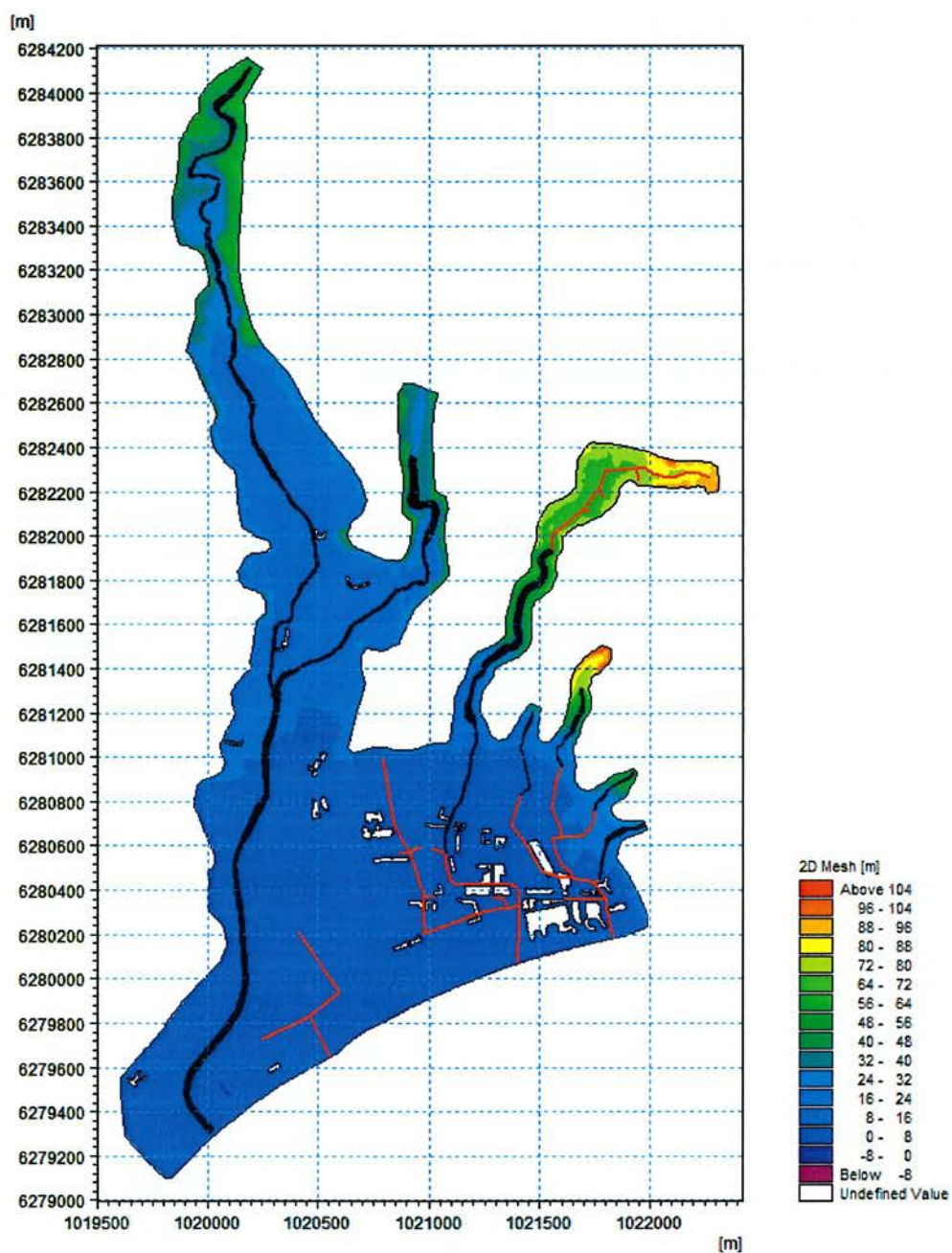
Figure 40 : Vue globale du modèle de l'aval de la Frayère, de la Roquebilière et du Devens.
